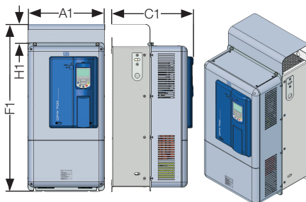
Frame size E up to 150 A with Nema1 kit Tamaño E hasta 150 A con kit Nema1 Mecânica E até 150 A com kit Nema1
