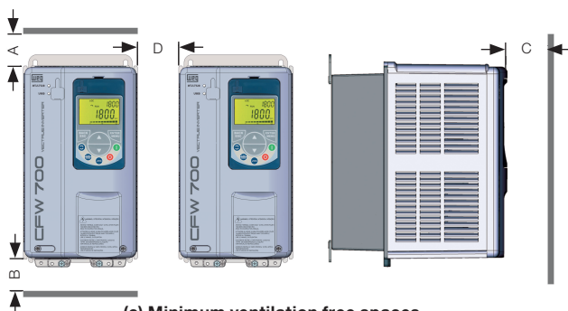
(c) Minimum ventilation free spaces (c) Espacios libres mínimos para ventilación (c) Espaços livres mínimos para ventilação
