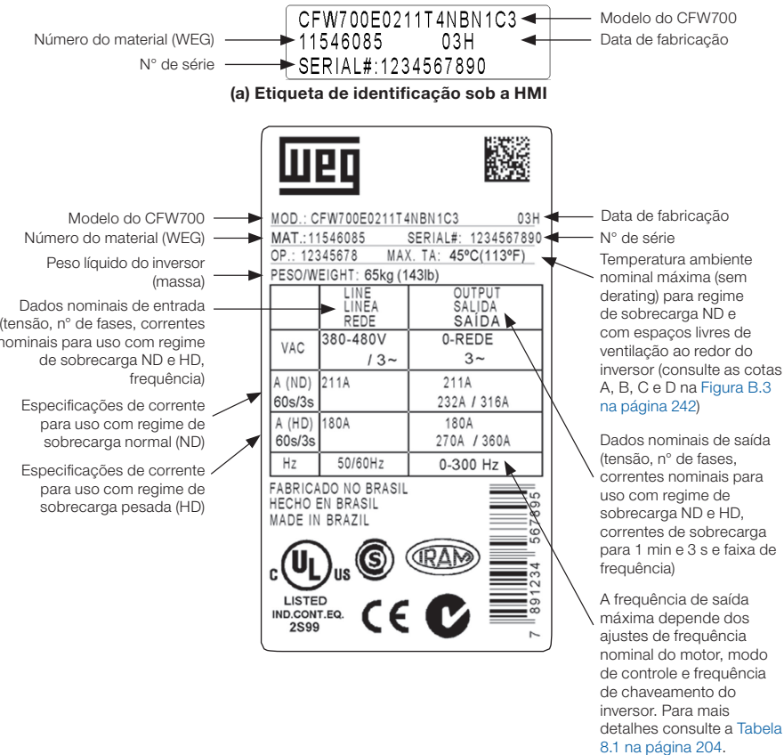
Figura 2.2: (a) e (b) Etiquetas de identificação
