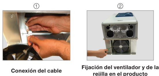
Figura 6.2: (a) y (b) Instalación del ventilador del disipador
