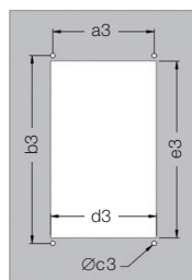
(b) Flange mounting - standard inverter (b) Montaje en flange - convertidor estándar (b) Montagem em flange - inversor padrão
