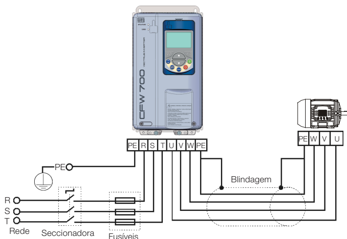
Figura 3.2: Conexões de potência e aterramento
