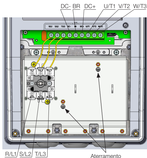
(b) Mecânicas B e C com grau de proteção IP55 e seccionadora
