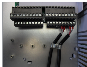
(b) Exemplo de ligação da blindagem ao terra
