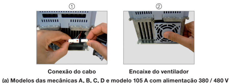
Figura 6.1: (a) e (b) Retirada do ventilador do dissipador
