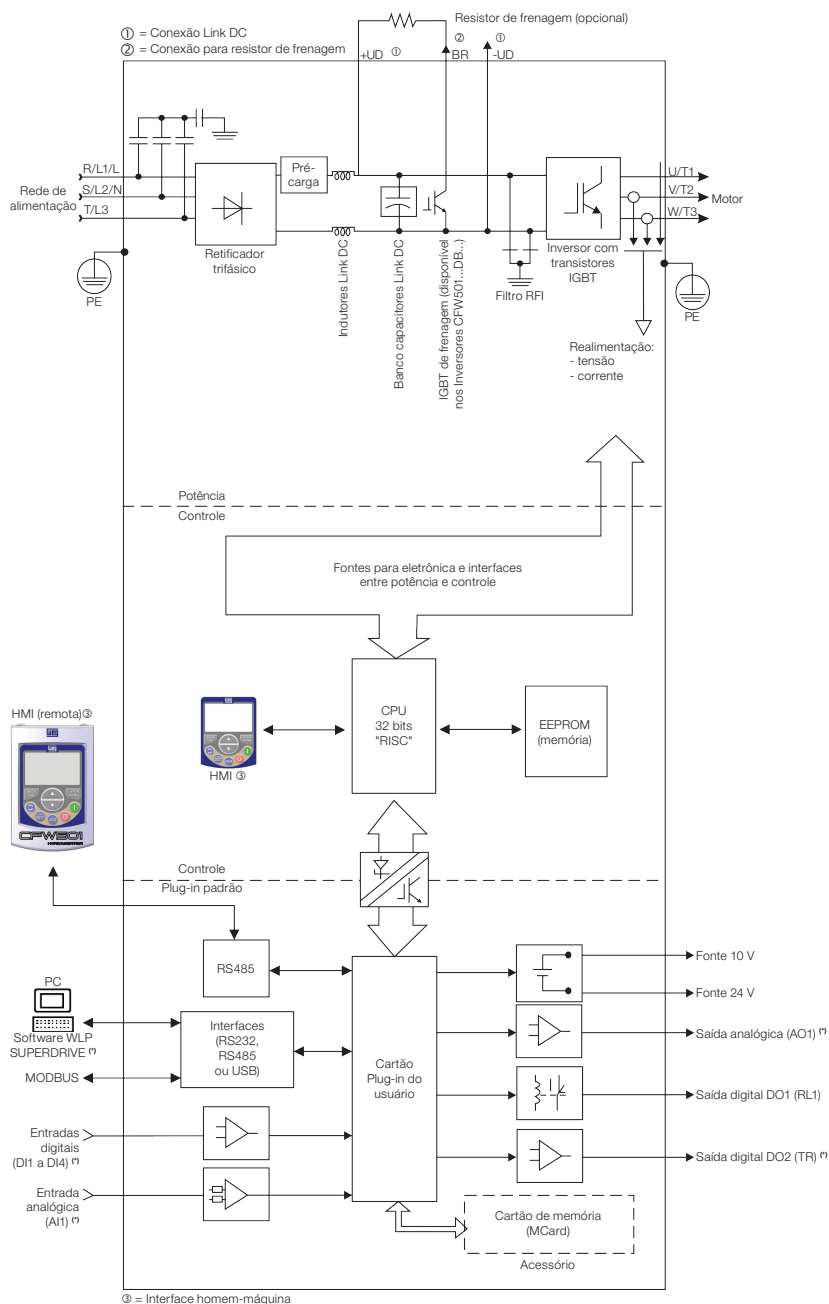
Figura 2.3: Blocodiagrama do CFW501 para mecânicas F e G
