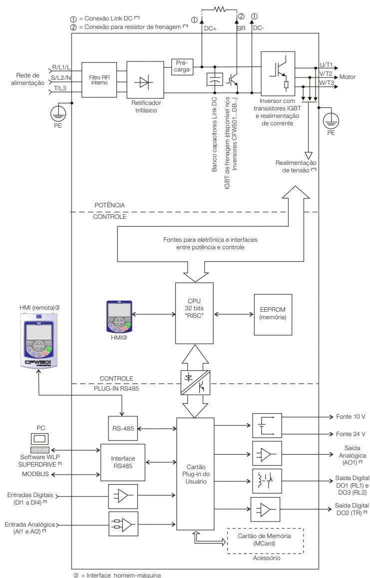
Figura 2.1: Blocodograma do CFW501 para mecânicas A, B e C
