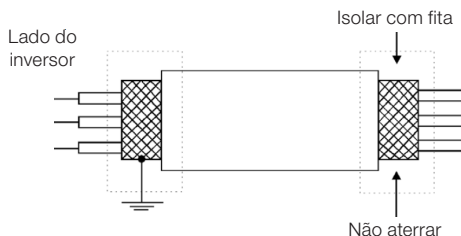
Figura 3.5: Conexão da blindagem
