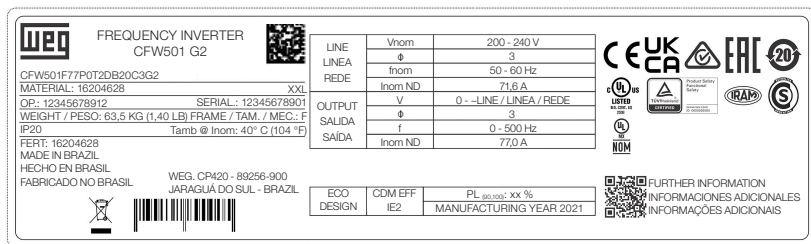
(b) Etiqueta lateral do CFW501 - mecânicas F e G
