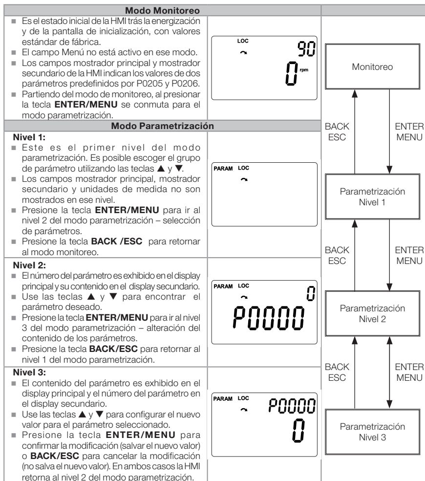
Figura 4.3: Modos de operación de la HMI
