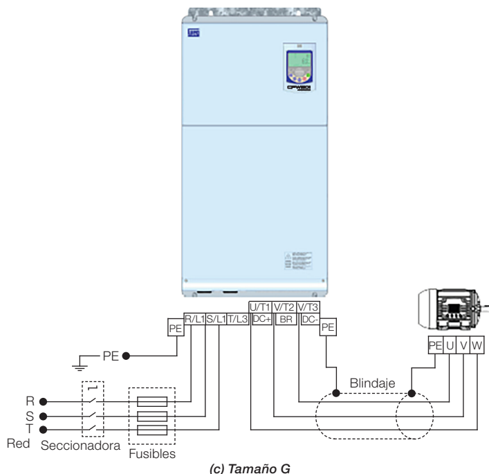
Figura 3.1: (a) to (c) Conexiones de potencia y aterramiento
