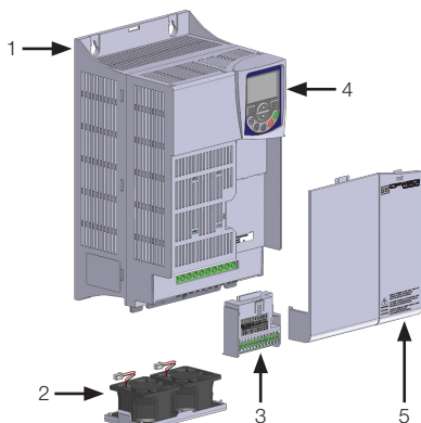
Frame Sizes D and E Tamaños D y E Mecânicas D e E
