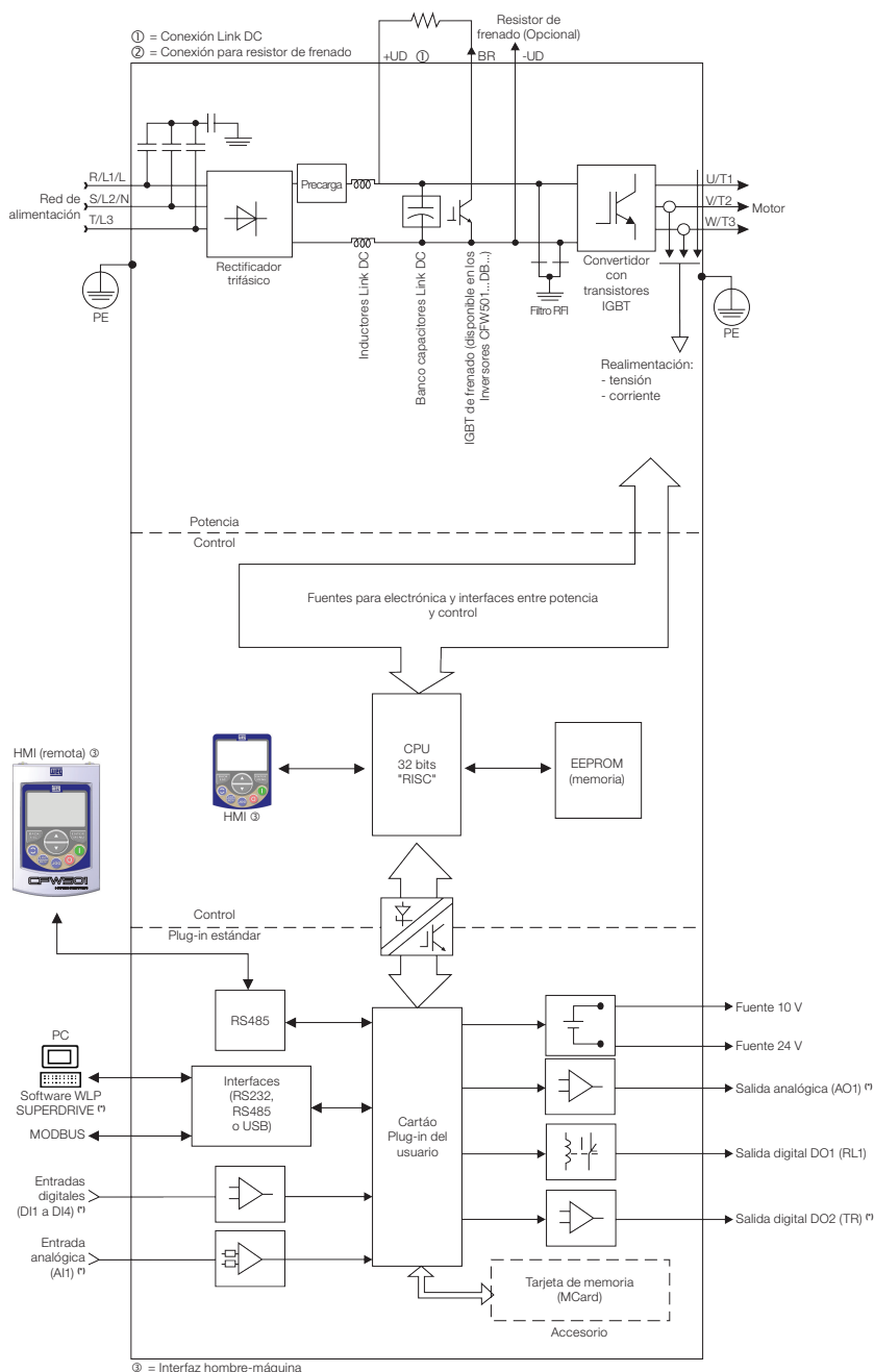
Figura 2.3: Diagrama de bloques del CFW501 para los tamaños F y G
