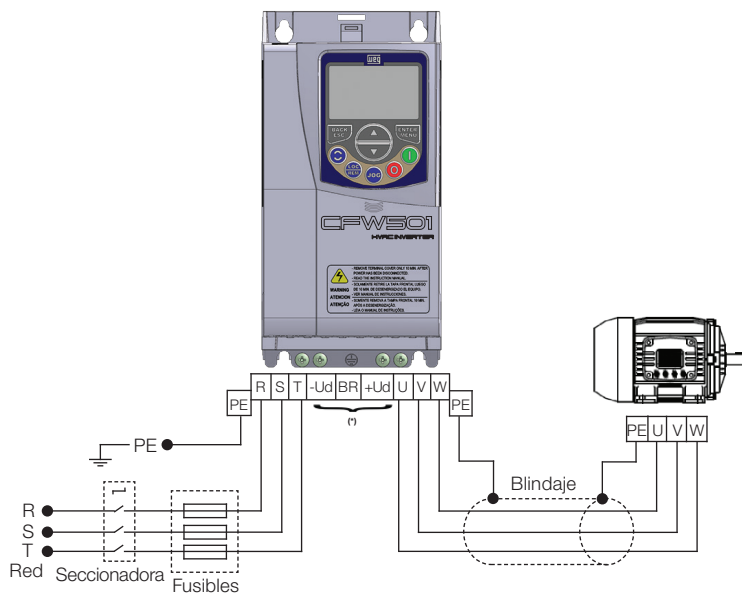
(a) Tamaños A, B, C y F
