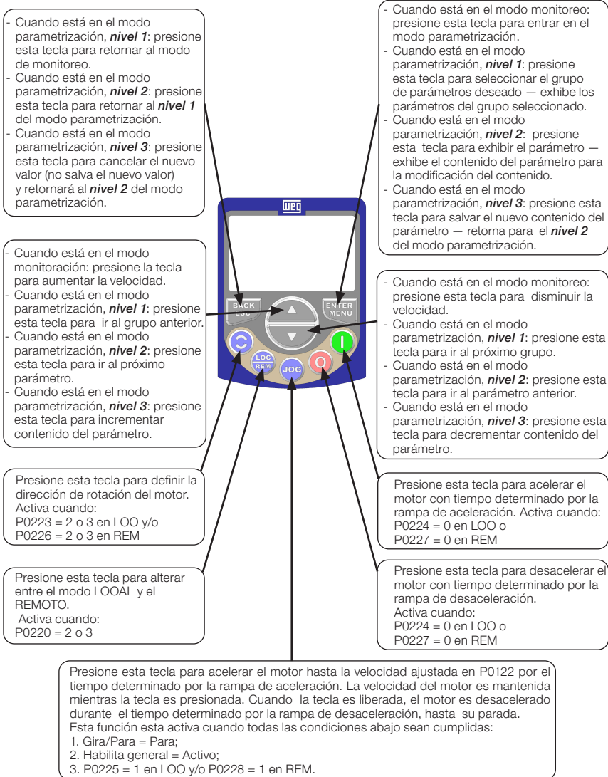
Figura 4.1: Teclas de la HMI
