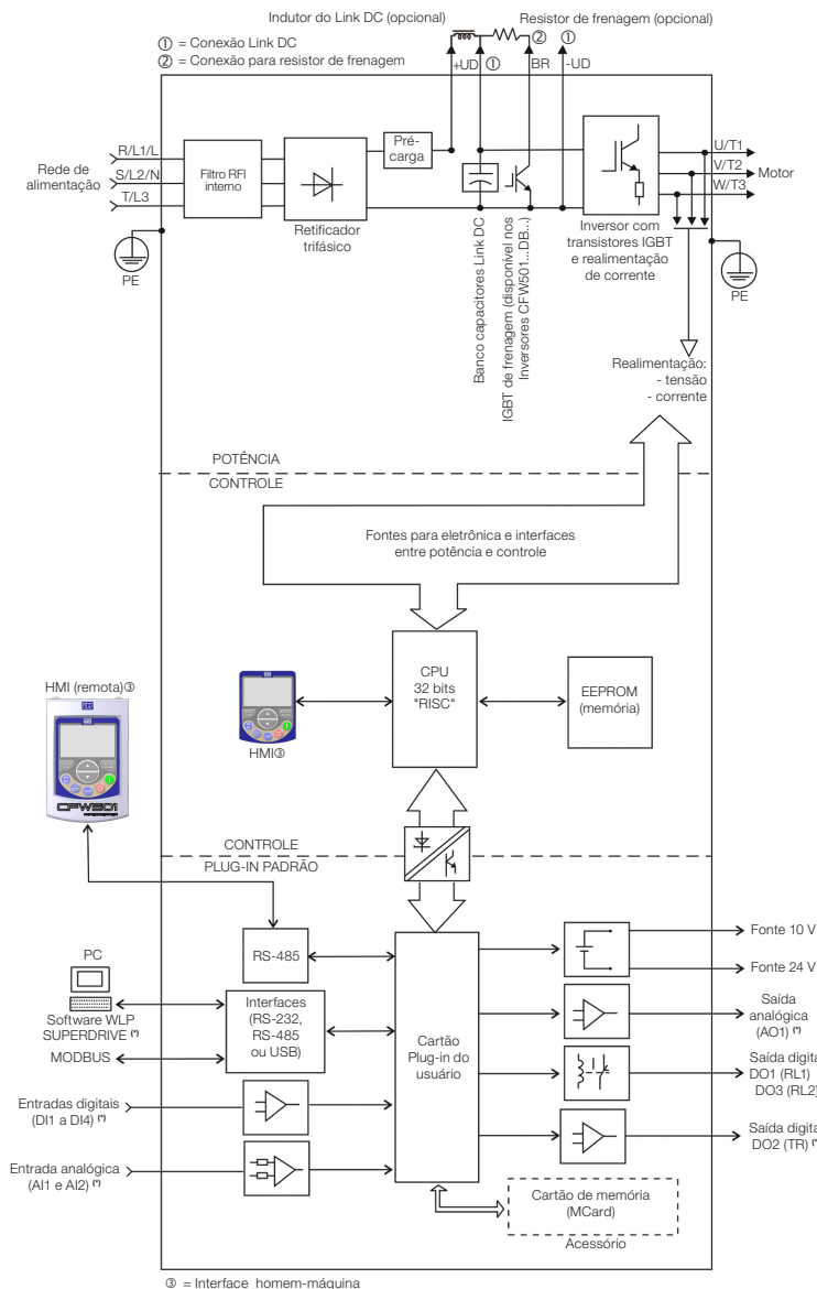
Figura 2.2: Blocodiagrama do CFW501 para mecânicas D e E
