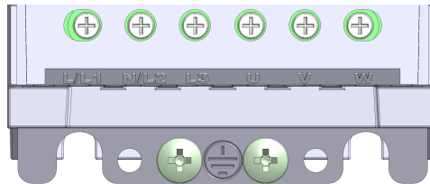
Frame Size A / Tamaño A / Mecânica A
