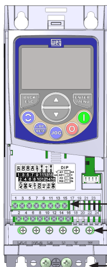
Frame size A Tamaño A Mecânica A
