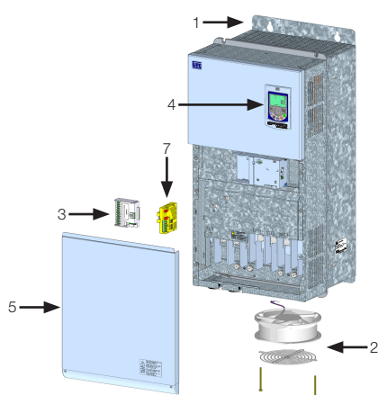
Frame Size G Tamaño G Mecânica G
