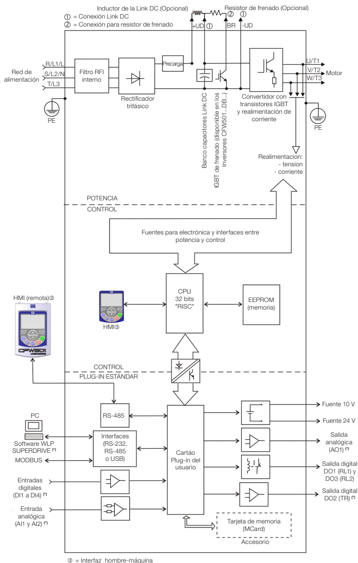
Figura 2.2: Diagrama de bloques del CFW501 para los tamaños D y E
