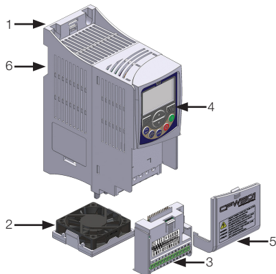
Frame Size F Tamaño F Mecânica F
