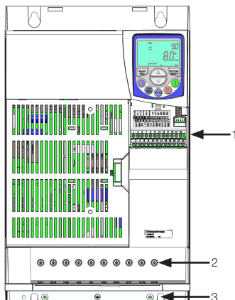
Frame Size E Tamaño E Mecânica E
