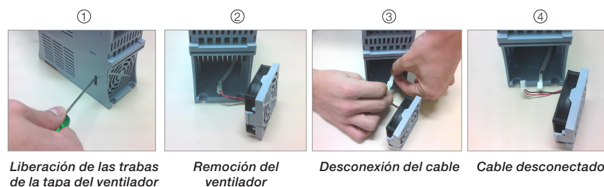
Figura 6.1: Retirada del ventilador del disipador
