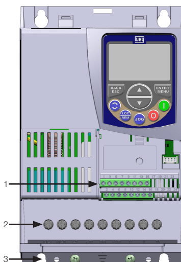
Frame size C Tamaño C Mecânica C
