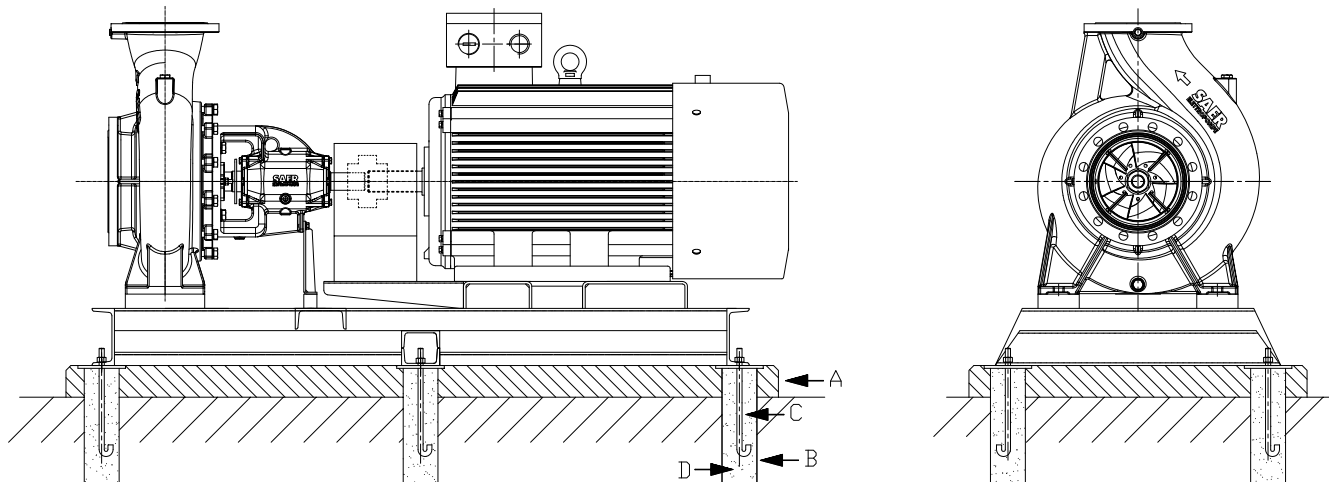
FIG. 7 Fissaggio del gruppo al suolo / Ground fixing of the group / Сбо́ре крепится к земле
